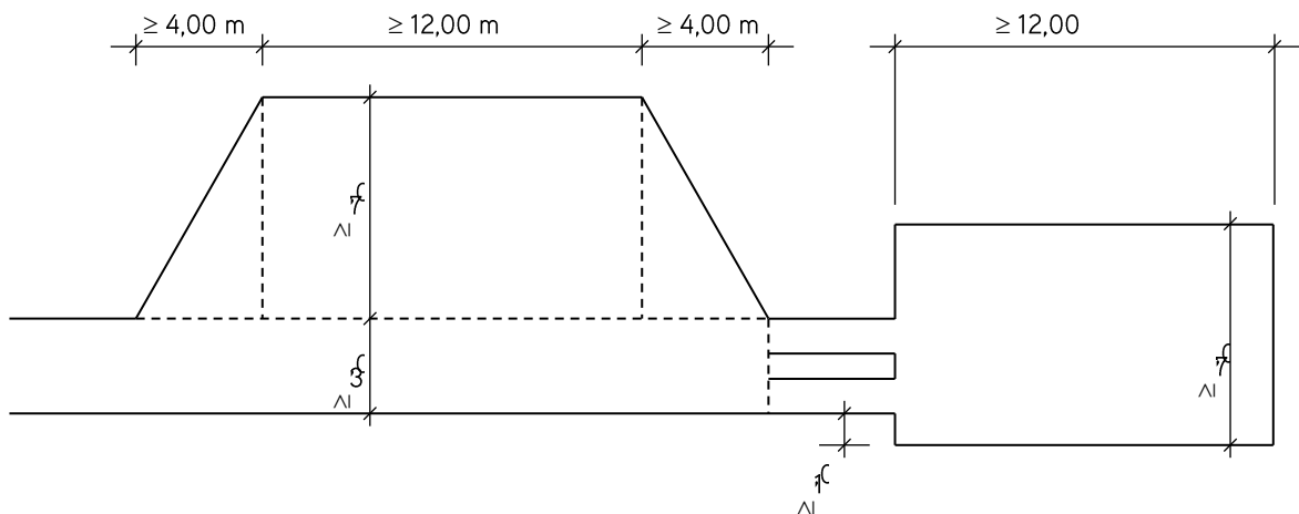
Bild 7 – Bewegungsflächen –
