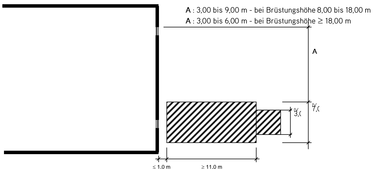
Bild 6 - Aufstellfläche rechtwinklig zur Außenwand
