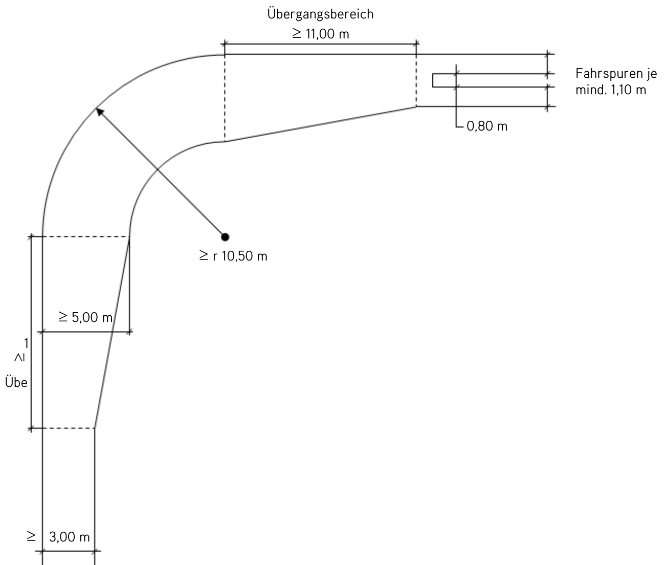
Bild 3 – nicht geradling geführte Zufahrt
