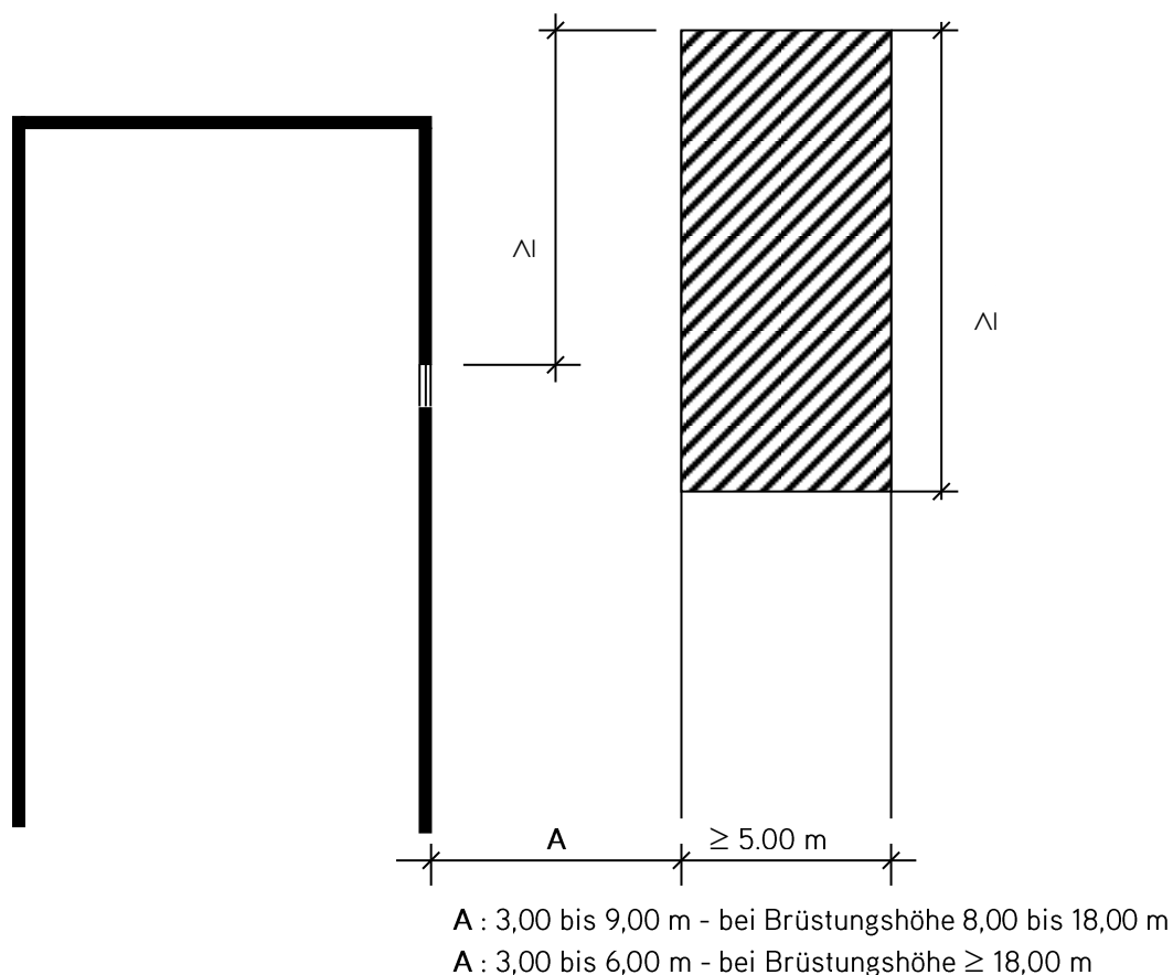
Bild 5 - Aufstellfläche entlang der Außenwand
