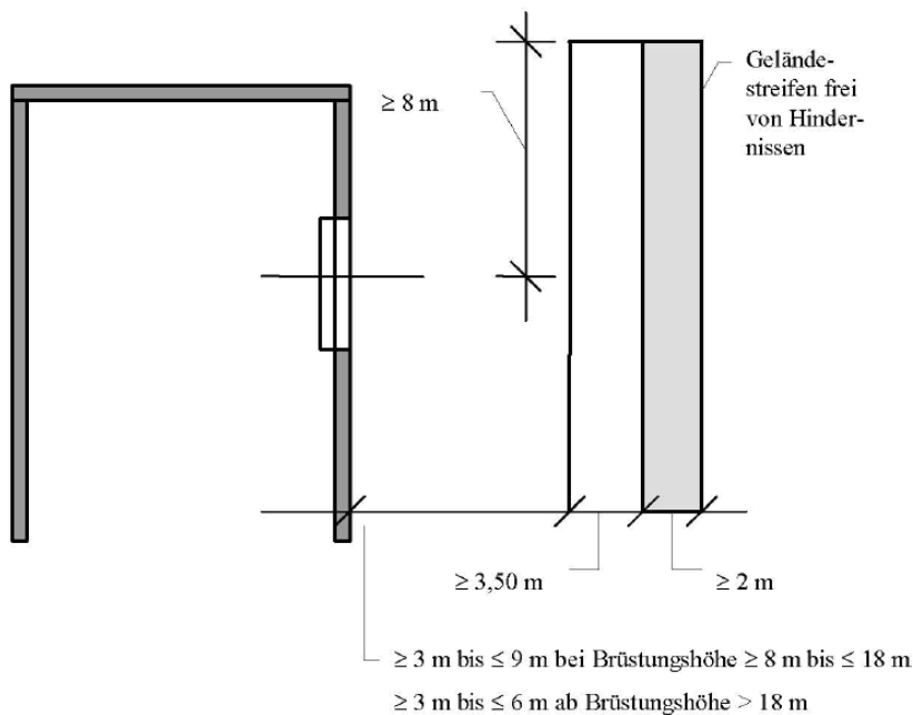
Bild 2 - Aufstellfläche entlang der Außenwand
