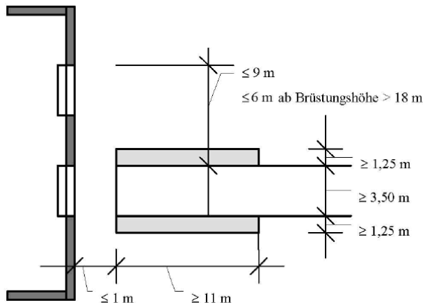
Bild 3 - Aufstellfläche rechtwinklig zur Außenwand
