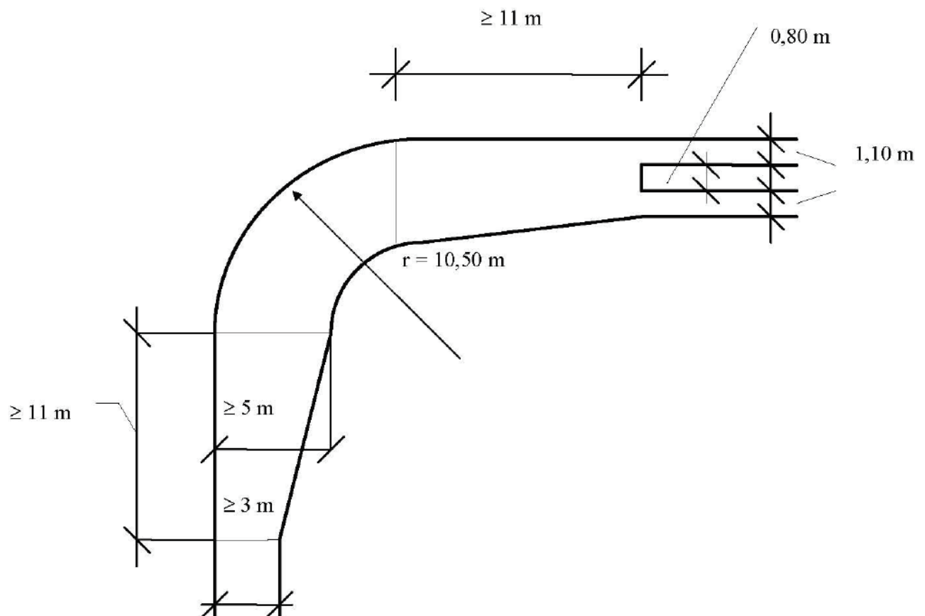
Bild 1 – nicht geradling geführte Zufahrt
